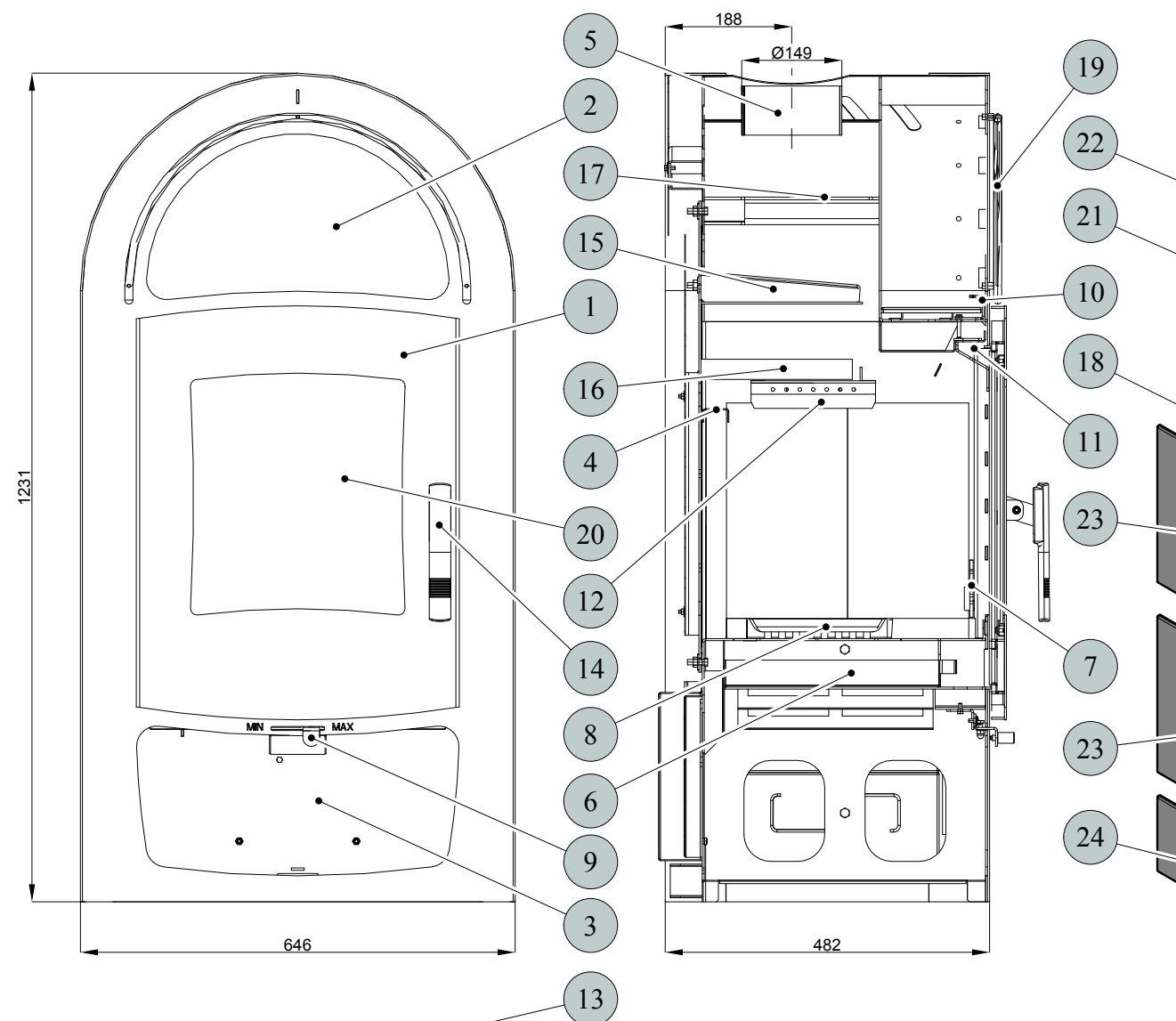
Informativní rozměr topeniště
