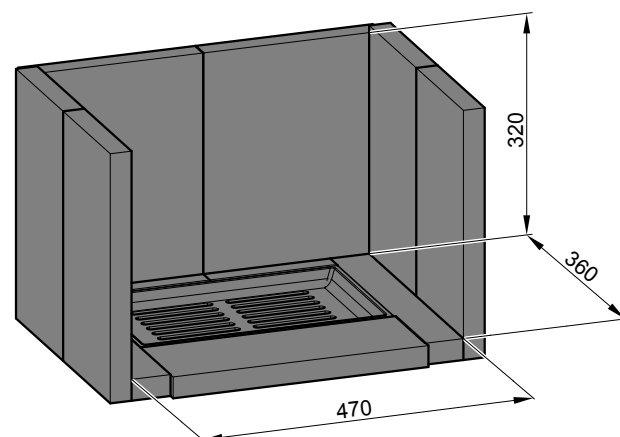
Informativní rozměr topeniště
